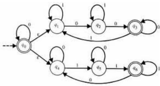
FSA
